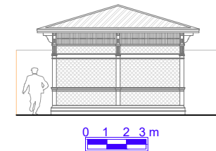
Elevação 04
