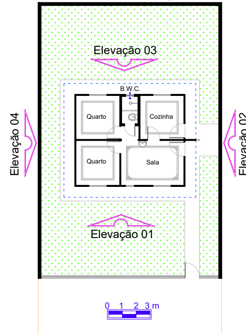
Planta
