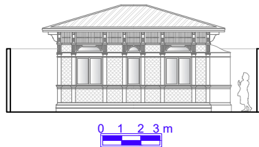
Elevação 01
